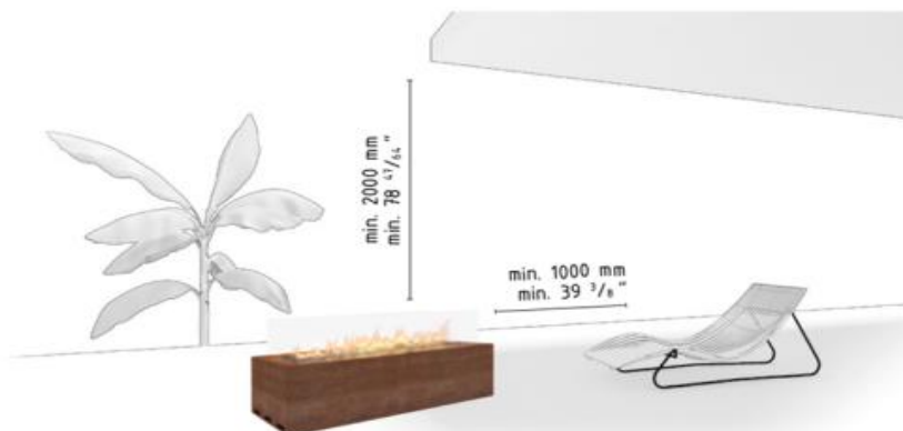
Abbildung 1: Mindestabstand zu brennbaren Materialien
